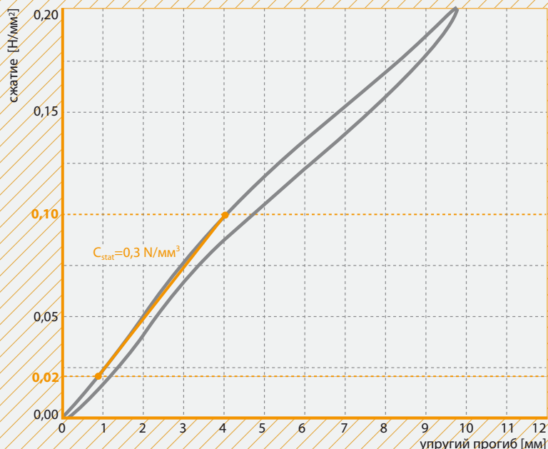
Кривая упругости подбалластного мата Sylodyn® DN 335
